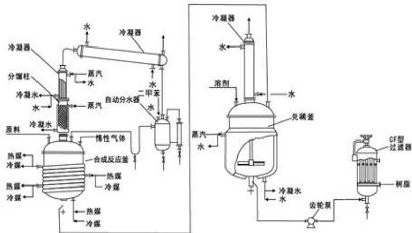
典型树脂生产流程
